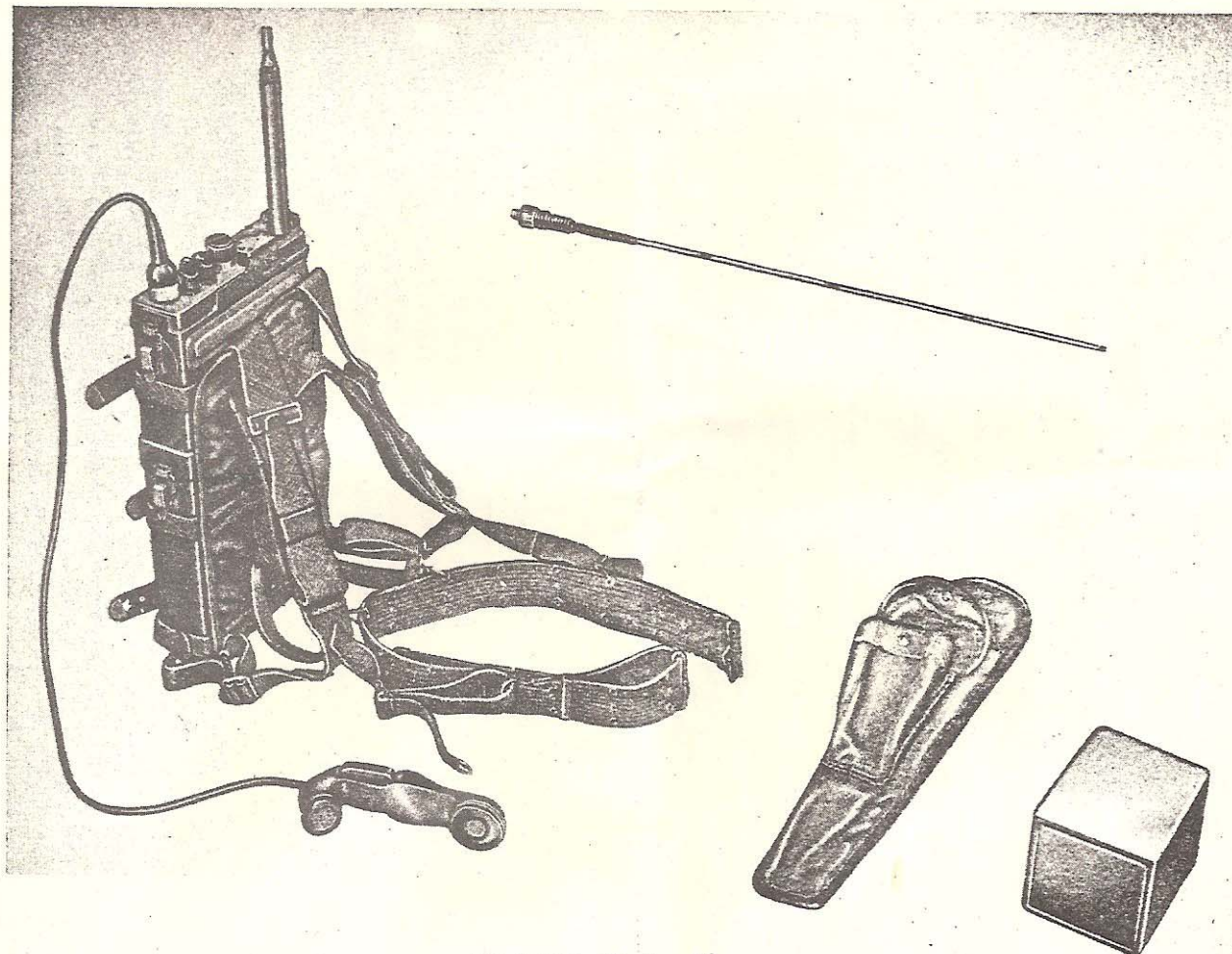
Fig. 1 - Stazioni AN/PRC - 8 ,9 e 10 .
